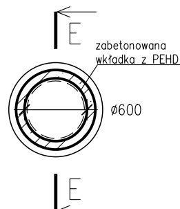
PRZEKRÓJ D-D
