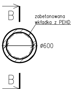
PRZEKRÓJ A-A
